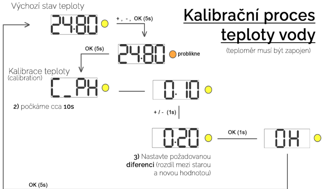
Obr 7 - průběh kalibračního procesu teploty
